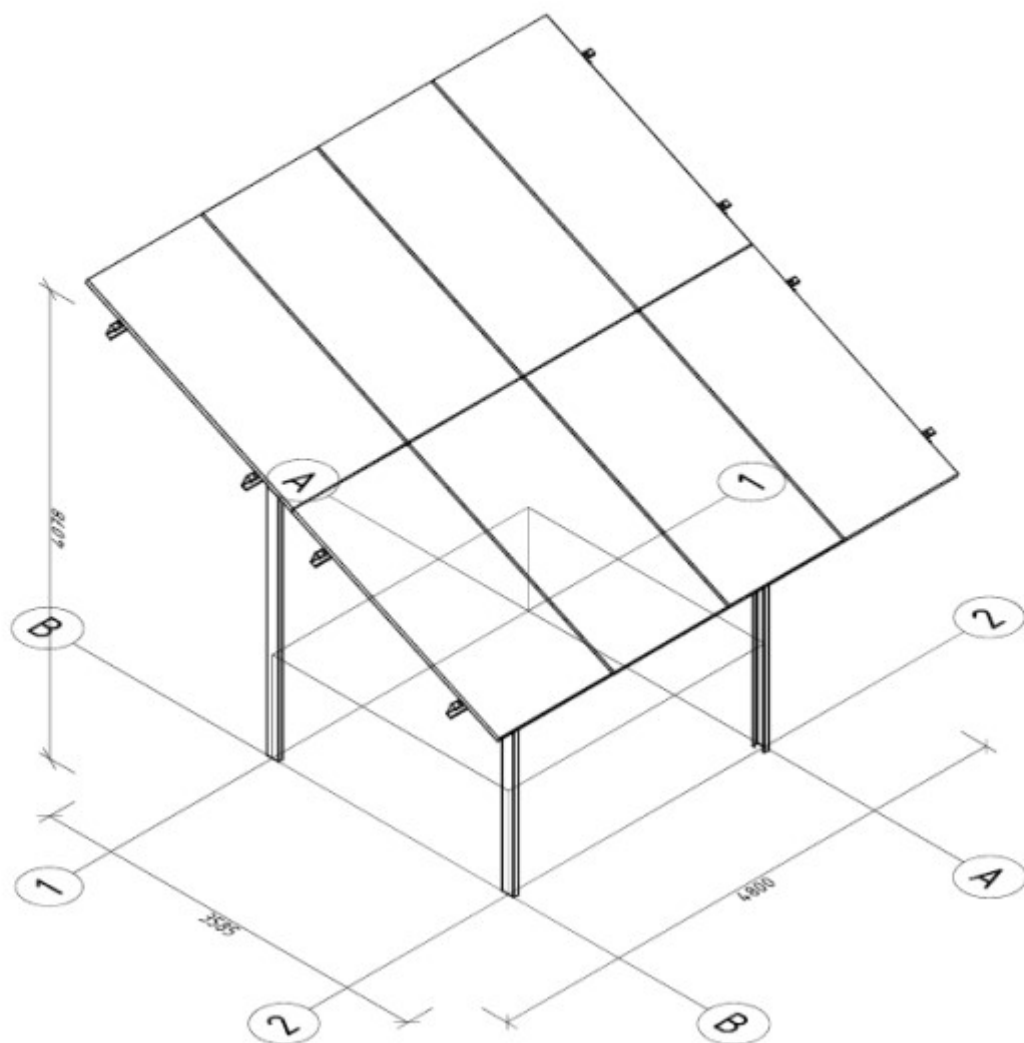
Wariant 1 Izometria NE 1#50 skala 1:50
